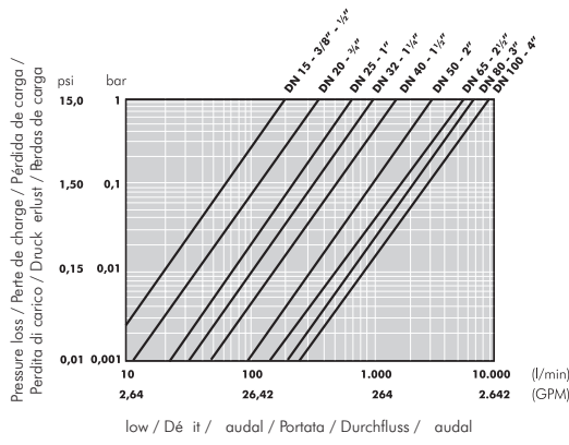
Pressure loss diagram Diagramme de perte de charge Diagrama de pérdidas de carga Diagramma delle perdite di carico Druckverlust-Diagramm Diagrama das perdas de carga
