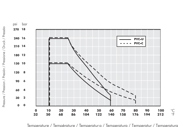
Pressure/temperature graph Diagramme pression/température Diagrama presión/temperatura Diagramma pressione/temperatura Druck-Temperatur-Diagramm Diagrama de pressão/temperatura
