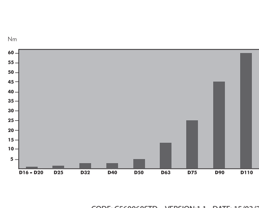
Torque graph Diagramme de couple Diagrama de par Diagramma di coppia Drehmoment-Diagramm Diagrama de par
